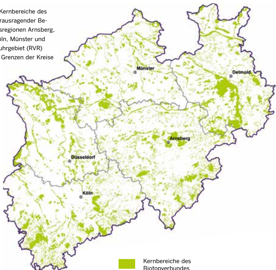
Abbildung 6: Kernbereiche des landesweiten Biotopverbundes
