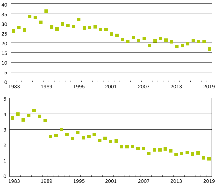
Abbildung 14: Indikator Stickstoff- und Säureeintrag
