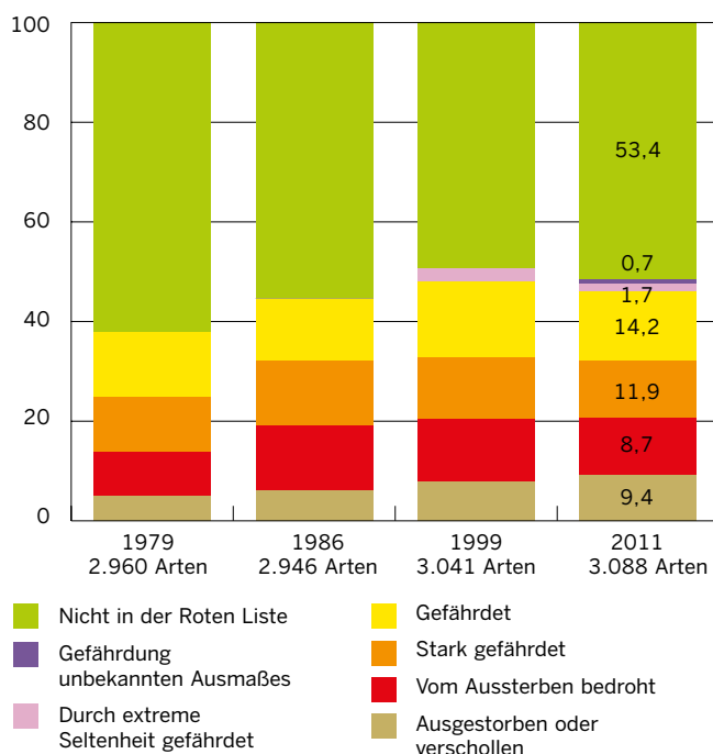
Abbildung 1: Gefährdete Arten (Angaben in %)
